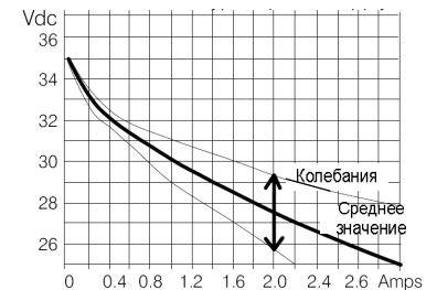
Диаграмма для типичного нерегулируемого источника питания
